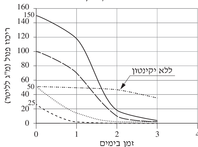
ריכוז פנול במכלי מים שונים שבהם גידלו צמחי יקינטון המים
